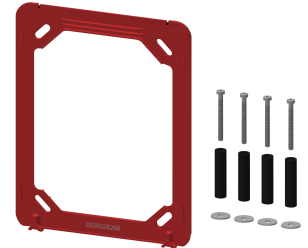
Halterahmen
