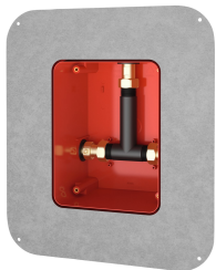
R5 Puszka systemowa do podtynkowych baterii z mieszaczem
