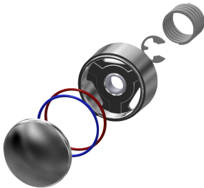
Druckkappe 2030042960 ASSV2001
